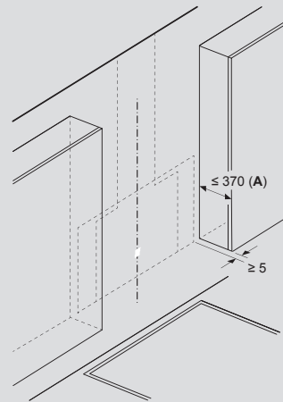
Gerät im Umluftbetrieb ohne Abluftkanal
