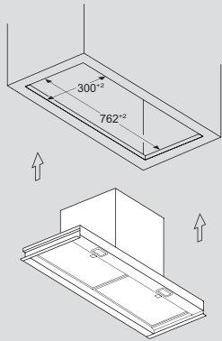
Einbaubeispiel in Möbelausschnitt
