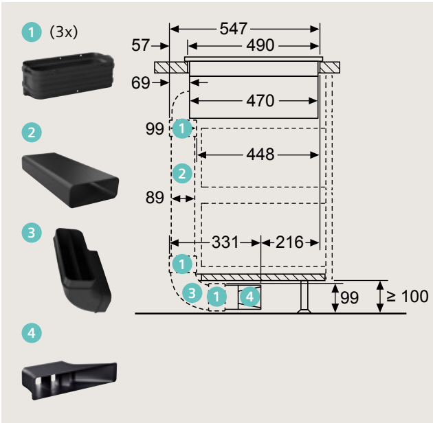
Verrohrungs-Set HZ9VDKR2 UHP € 150,-**
