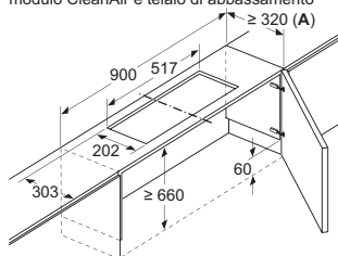
Montaggio cappa a schermo piatto con modulo CleanAir e telaio di abbassamento
