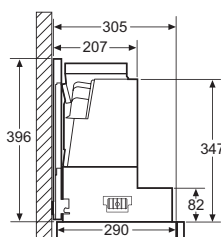
Montaggio apparecchi con telaio di abbassamento - Profondità del mobile secondo la tabella delle combinazioni
