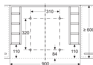
Montaggio cappa a schermo piatto con telaio di abbassamento Mobili con ripiani laterali Montaggio diretto sulla parete della cucina
