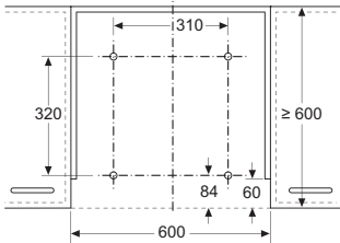
Montaggio cappa a schermo piatto con telaio di abbassamento Montaggio diretto sulla parete della cucina
