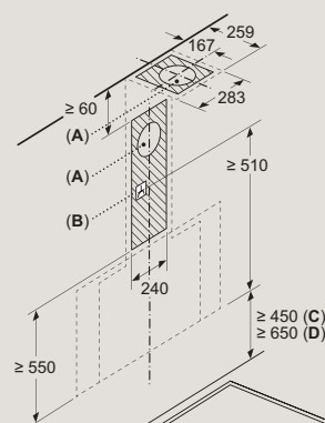
Installazione a parete con camino
