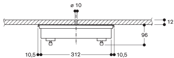
Sección transversal
