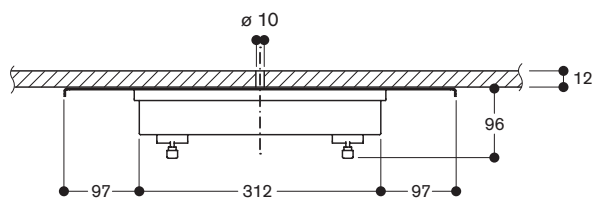
Sección transversal
