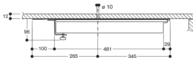
Sección longitudinal
