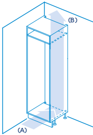
A: Entrada de aire ≥ 200 cm²; opciones de ventilación B: Salida de aire ≥ 200 cm²; opciones de ventilación
