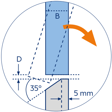
Instalación con achaflanado interior del cajón
