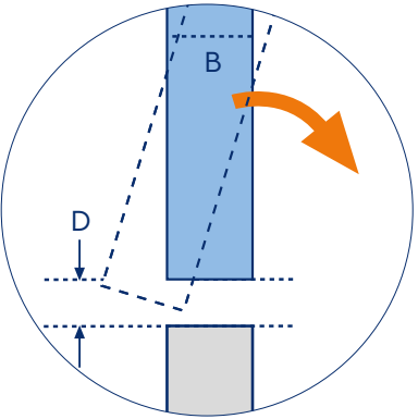
Instalación sin achaflanado interior del cajón
