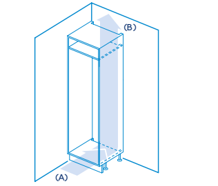
A: Entrada de aire ≥ 200 cm²; opciones de ventilación B: Salida de aire ≥ 200 cm²; opciones de ventilación
