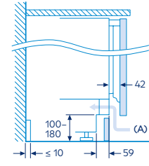
A: Entrada de aire ≥ 200 cm²
