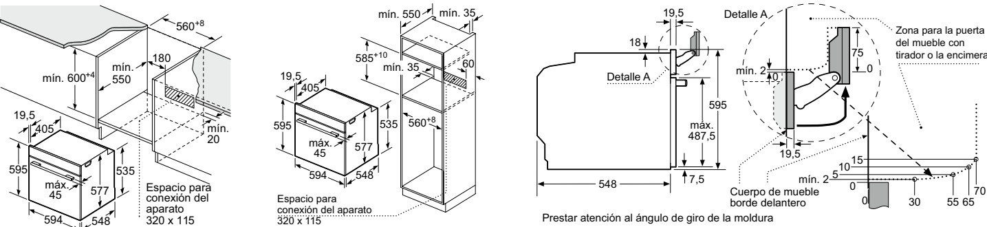
Dimensiones en mm
