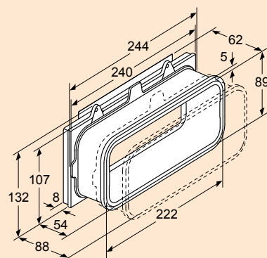
Złączka wyposażenie „Plug 'n Play” przystosowują- ce wyciąg do pracy w obiegu zamkniętym.
