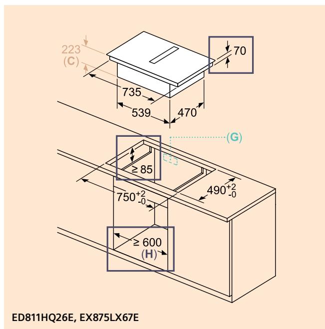
inductionAir Plus instalacja na blacie
