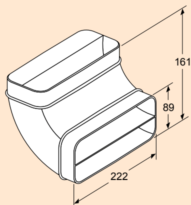
HZ9VDSB2 kolanko 90° „L”, kanał płaski, pionowy (część męska).
