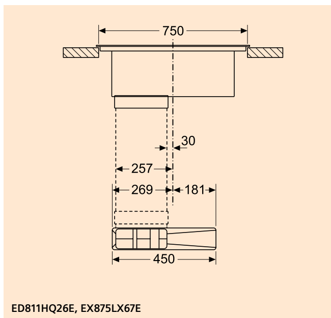
Widok z przodu: inductionAir Plus przy instalacji na blacie kuchennym
