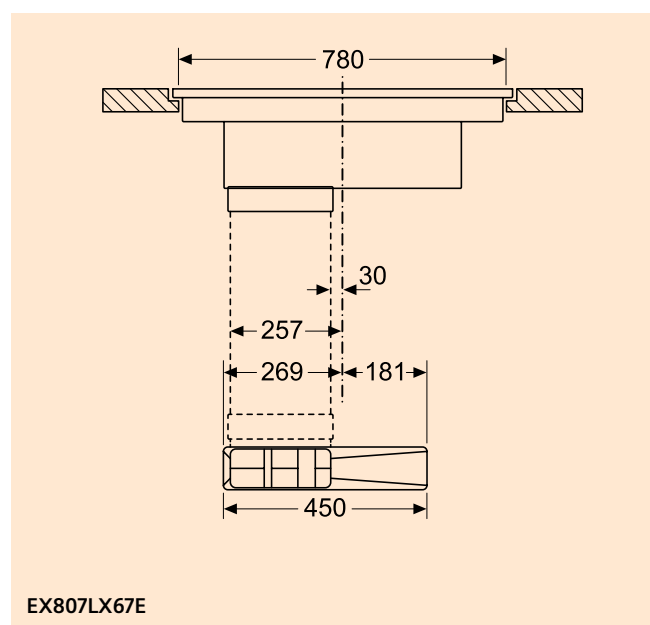
Widok z przodu: inductionAir Plus przy instalacji na równi z blatem kuchennym
