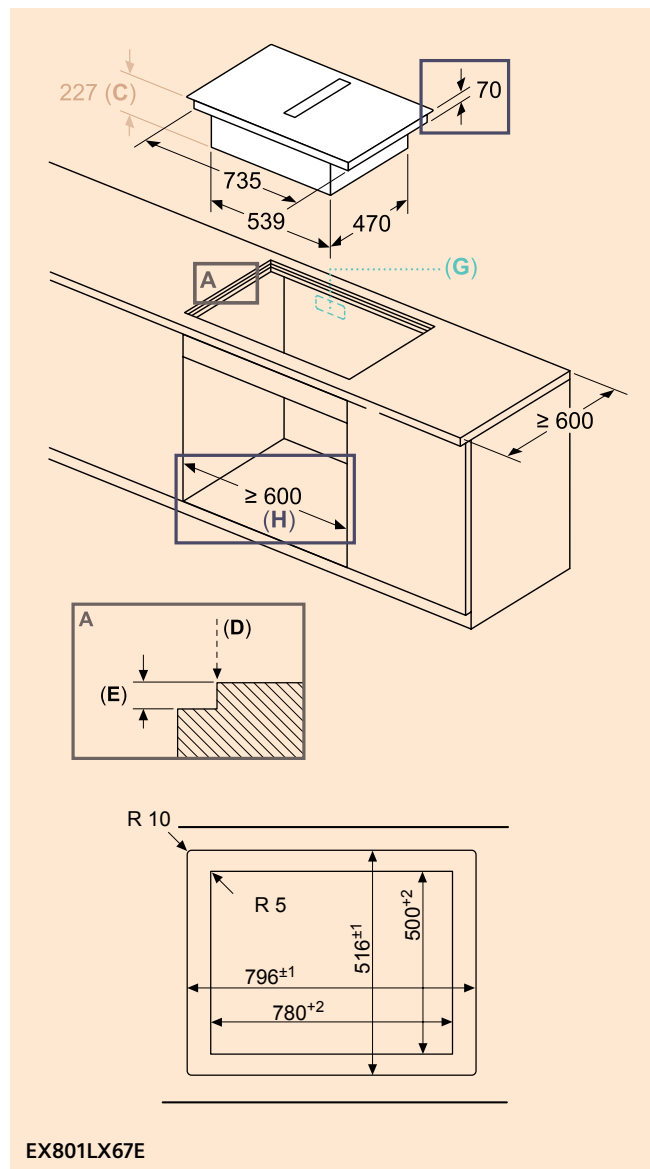
inductionAir Plus instalacja na równi z blatem
