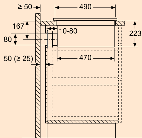
inductionAir Plus montaż na blacie ED811HQ26E
