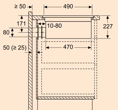
inductionAir Plus montaż na równi z blatem EX801LX67E
