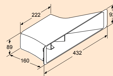
HZ9VRPD1 Dyfuzor wyposażenie przystosowujące wyciąg do pracy w obiegu zamkniętym z pełnym lub częściowym odprowadze- niem kanałowym.
