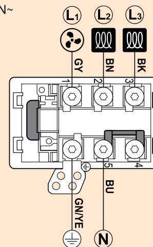
Przykładowy schemat połączeń elektrycznych dla prądu 3-fazowego.
