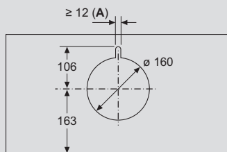
A: Passage de câbles
