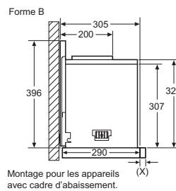
Montage d'une hotte plate avec cadre d'abaissement Meuble avec étagères latérales Montage directement contre le mur de la cuisine
