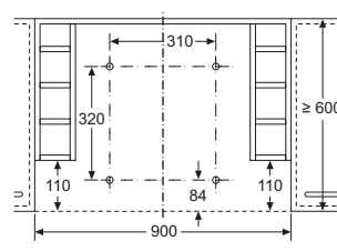
Montage d'une hotte plate avec cadre d'abaissement Meuble avec étagères latérales Montage directement contre le mur de la cuisine
