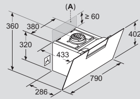
Appareil en mode circulation d'air sans conduit
