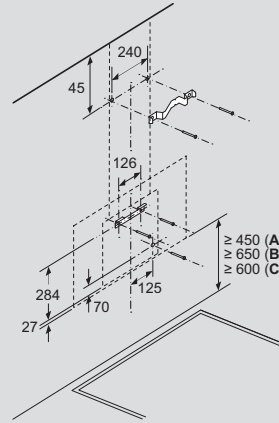
Installation murale avec cheminée
