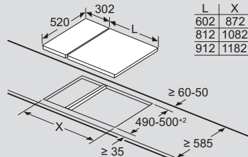
Einbaubeispiel für Montagesatz 1 Domino-Kochfeld + 1 Kochfeld
