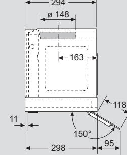
Seitenansicht
