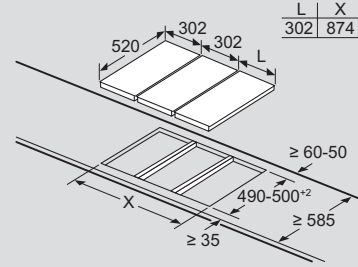
Einbaubeispiel für Montagesatz 3 Domino-Kochfelder
