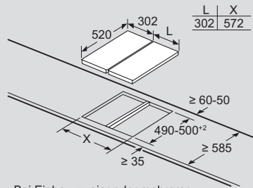
Einbaubeispiel für Montagesatz 2 Domino-Kochfelder
