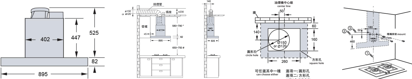
安裝圖 Installation diagrams
