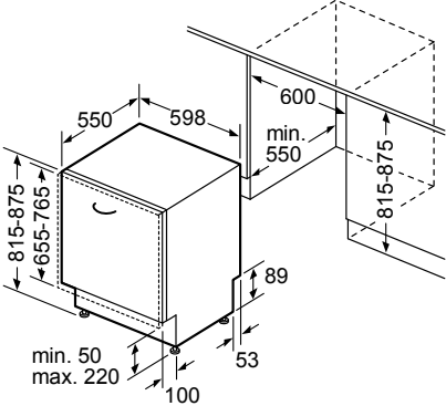
SN-modellen met varioScharnier
