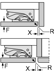
Afmeting in mm Aanbeveling tussenruimtes voor vlakscharnier
