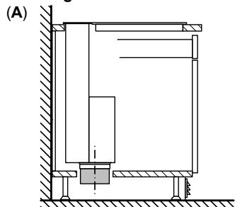
A: Buitenwand – U-waarde \leq 0,5 \text{ W/(m}^2\text{K)}
