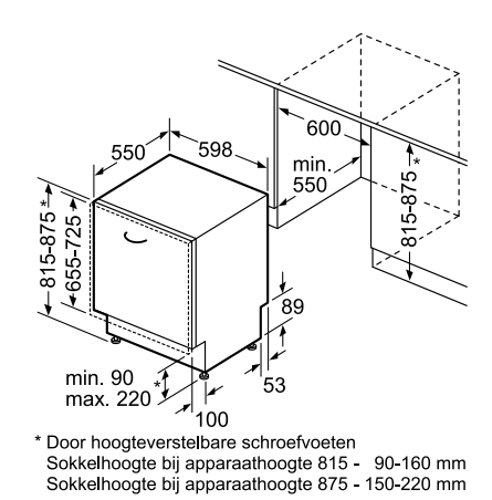
SN-modellen zonder varioScharnier
