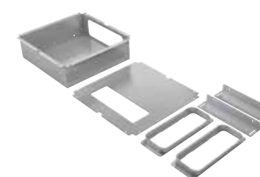
LZ29IDP00 Aktivt kullfilter startsett – Long Life Startsett for aktivt kullfilter. Aktivt kullfilter. Estimert levetid: 12 måneder. Redusering av mato: > 80 %. Regenereringsprosess: 2 timer på 200 °C i ovnen hver fjerde måned. Inneholder sett med 2 kullfiltere, 2 monteringsrammer og ventilatorrør. Veil. pris kr. 3 004
