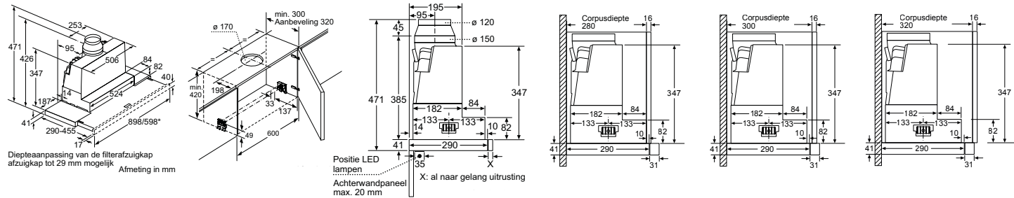
Afmeting in mm
