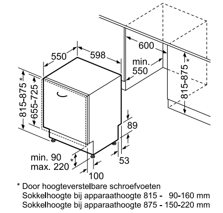
SN-modellen zonder varioScharnier Maten in mm
