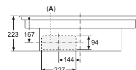
Afmeting in mm Vooraanzicht
