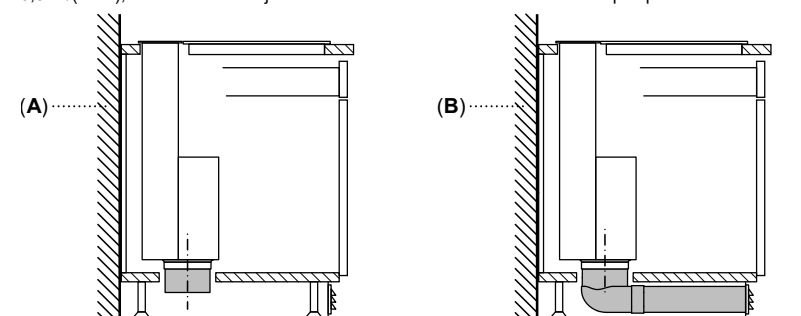
A: Buitenmuur – U-waarden \leq 0,5 \text{ W/(m}^2\text{K)} B: Buitenmuur – U-waarden >0,5 \text{ W/(m}^2\text{K)}
