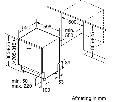
SX-modellen met varioScharnier
