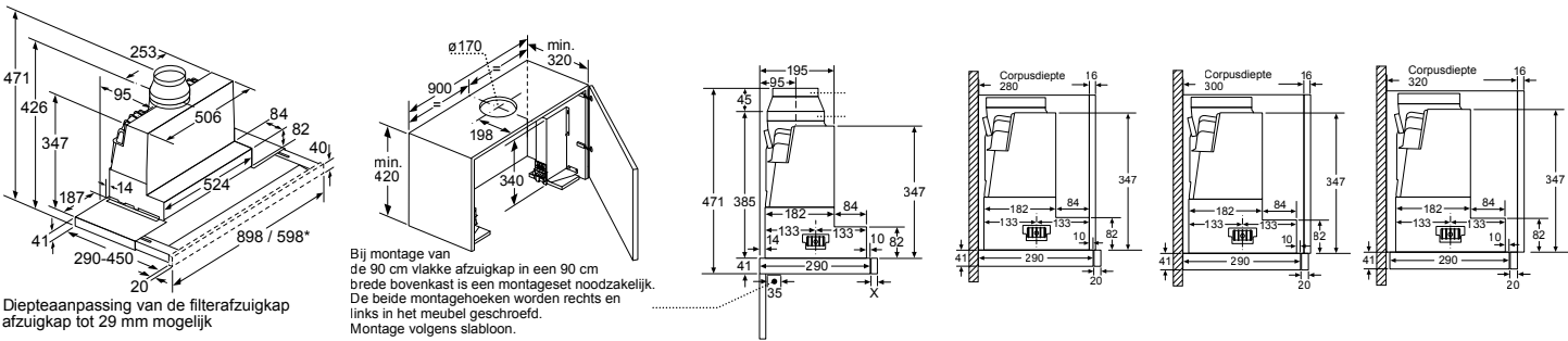
Afmeting in mm
