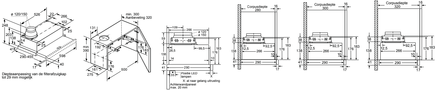
Afmeting in mm
