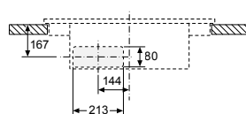
Afmeting in mm Vooraanzicht - Meubeluitsparing voor circulatielucht zonder kanaal
