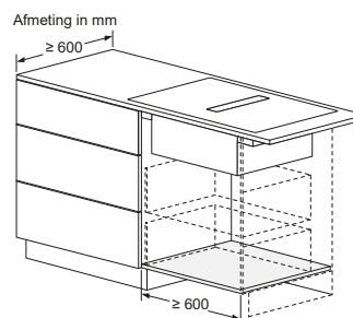
Afmeting in mm Vooraanzicht - Meubeluitsparing voor circulatielucht zonder kanaal
