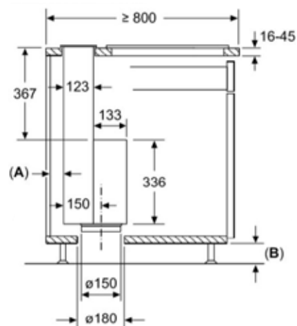
A: Ten minste 2 cm afstand van de Guided Air afzuiging/unit tot aan muur B: \geq 600 \text{ mm} bij recirculatie \geq 100 \text{ mm} bij recirculatie met bebuizing
