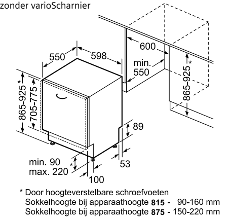
SX-modellen zonder varioScharnier Maten in mm
