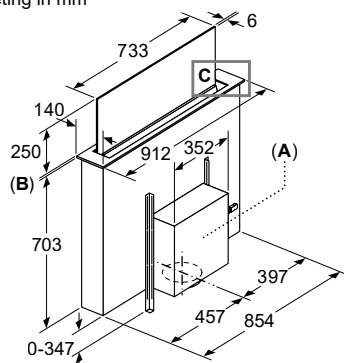
A: De motorunit kan worden gemonteerd aan de voorzijde of de achterzijde of op maximaal drie meter van het apparaat. (speciaal toebehoren noodzakelijk) B: 5.5
