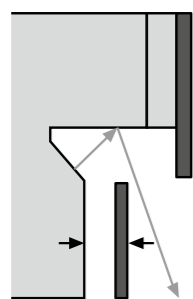
Retranqueo de zócalo mueble al lavavajillas (máx. 60)
