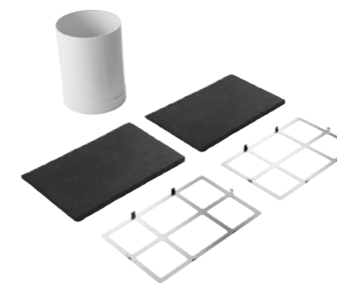
LZ29IDP00 Standard kulfiltersæt – Long Life Startsæt til brug for recirkulation. Standard kulfilter. Levetid: 12 måneder. Lugtreduktion: > 80 %. Regenereringsproces: 2 timer ved 200 °C i ovnen hver 4. måned. Indeholder 2 kulfiltre, fleksslange og 2 monteringsrammer. Vejl. pris kr. 2 072
