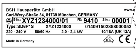
Beispiel des Typenschildes mit E-Nr. und FD
