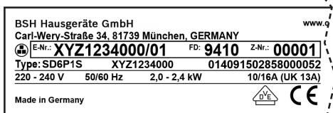
Ejemplo de placa de características con E-Nr y FD
