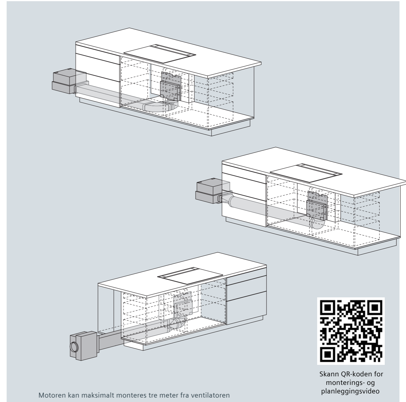
Eksempler på montering
