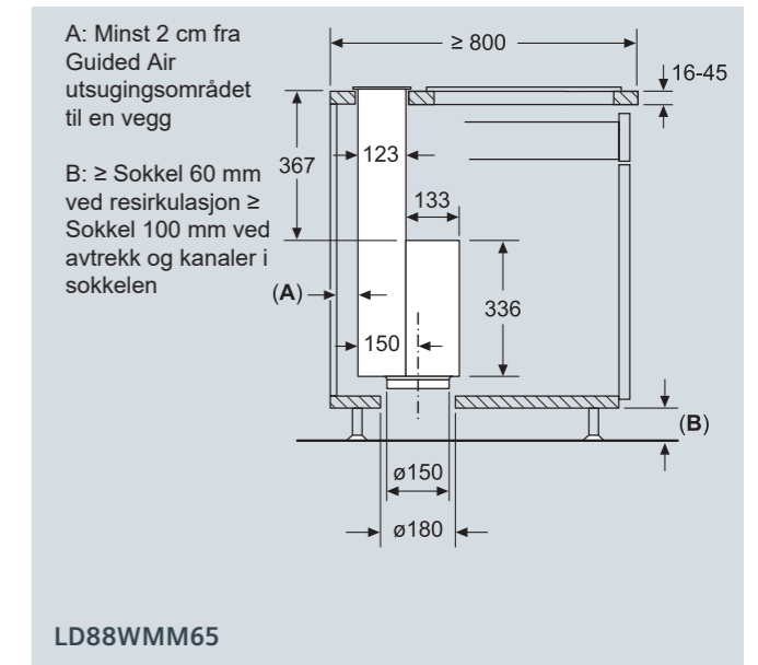
glassdraftAir - Mål sett fra siden ved separat montering av ventilator og platetopp
