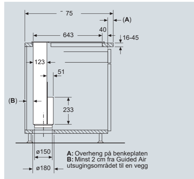
Ventilator med beslag sett fra siden ved montering av glidende overgang
