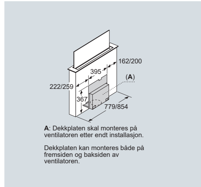
Ventilator med beslag sett fra siden ved montering av glidende overgang
