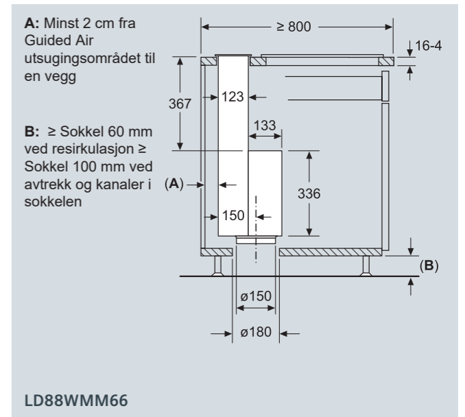
glassdraftAir - Mål sett fra siden ved separat montering av ventilator og platetopp
