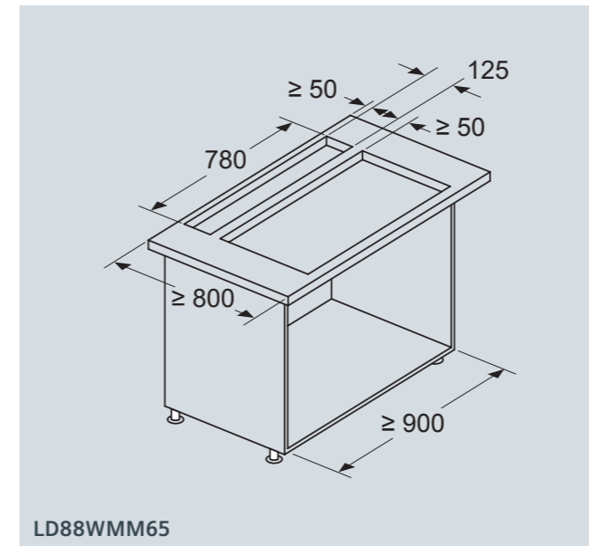
glassdraftAir - Utskjæringsmål ved separat montering av platetopp og ventilator.
