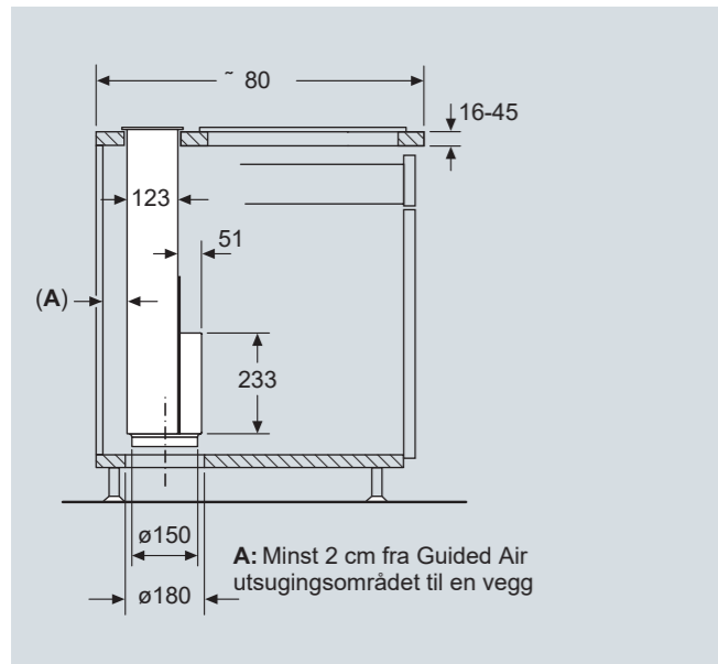
Ventilator med beslag sett fra siden ved separat montering av ventilator og platetopp
