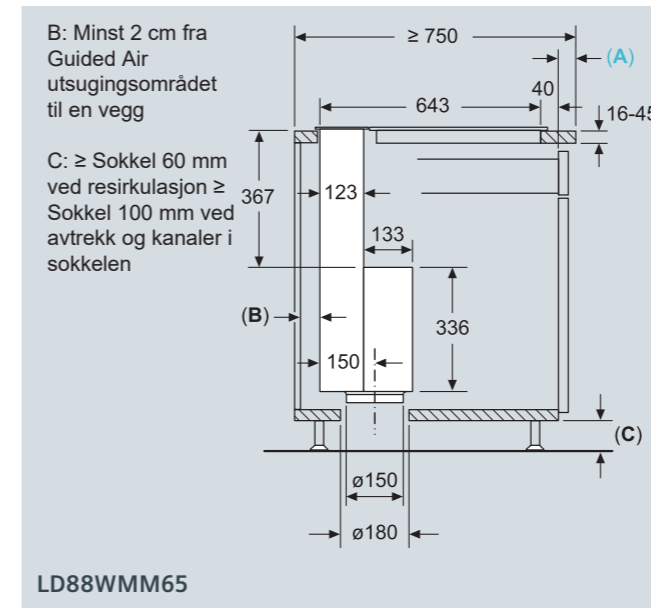
glassdraftAir - Mål sett fra siden ved separat montering av ventilator og platetopp
