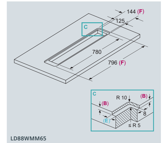
glassDraftAir (Uten ramme - planoDesign) utskjæringsmål til innbygging i stein og granittbenkeplater.
