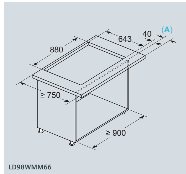
glassdraftAir - Utskjæringsmål til montering med glidende overgang (med monteringssettet LZ29WWY12)
