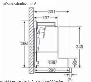
montáž pri spotrebičoch so spúšťacím rámom – hĺbka korpusu skrinky podľa tabuľky s kombináciami
