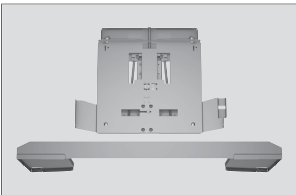
spôsob zabudovania spotrebiča v skrinke zabudovaná hĺbka spotrebiča so spúšťacím rámom hĺbka držadla (X) celková zabudovaná hĺbka hĺbka korpusu skrinky spôsob zabudovania A 301 17 318 ≥ 320 301 20 321 ≥ 323 301 31 332 ≥ 334 spôsob zabudovania B 301 31 332 ≥ 334
