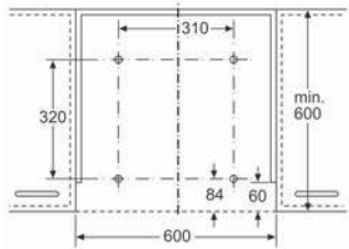
montáž spotrebiča so spúšťacím rámom | montáž priamo na kuchynskú stenu
