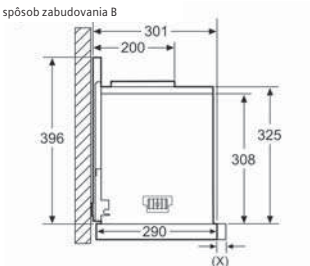
montáž pri spotrebičoch so spúšťacím rámom – hĺbka korpusu skrinky podľa tabuľky s kombináciami
