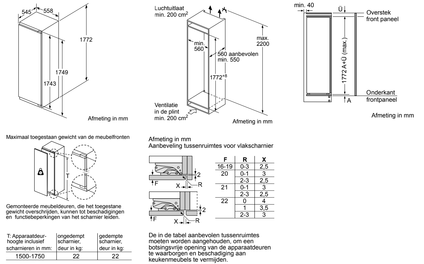
GI81NACF0 Afmetingen in mm
