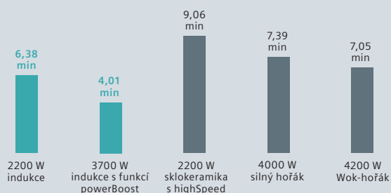
Čas potřebný pro ohřev 2 litrů vody o teplotě 15 °C na teplotu 90 °C (v minutách)
