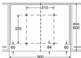
montáž spotřebiče se spouštěcím rámem montáž přímo na kuchyňskou zeď
