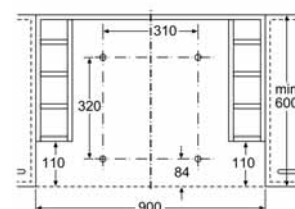
montáž spotřebiče se spouštěcím rámem skříňka s postranními policemi montáž přímo na kuchyňskou zeď
