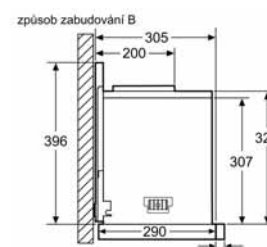
montáž u spotřebičů se spouštěcím rámem – hloubka korpusu skříňky podle tabulky s kombinacemi
