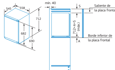
Dimensiones del espacio recomendadas para instalación de puerta fija
