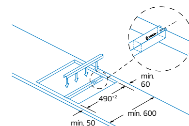
Accesorio de unión 3AB3030L
