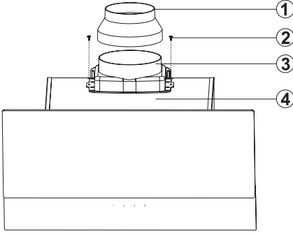
Res. 11: PLASTİK BACA BAĞLANTISI
