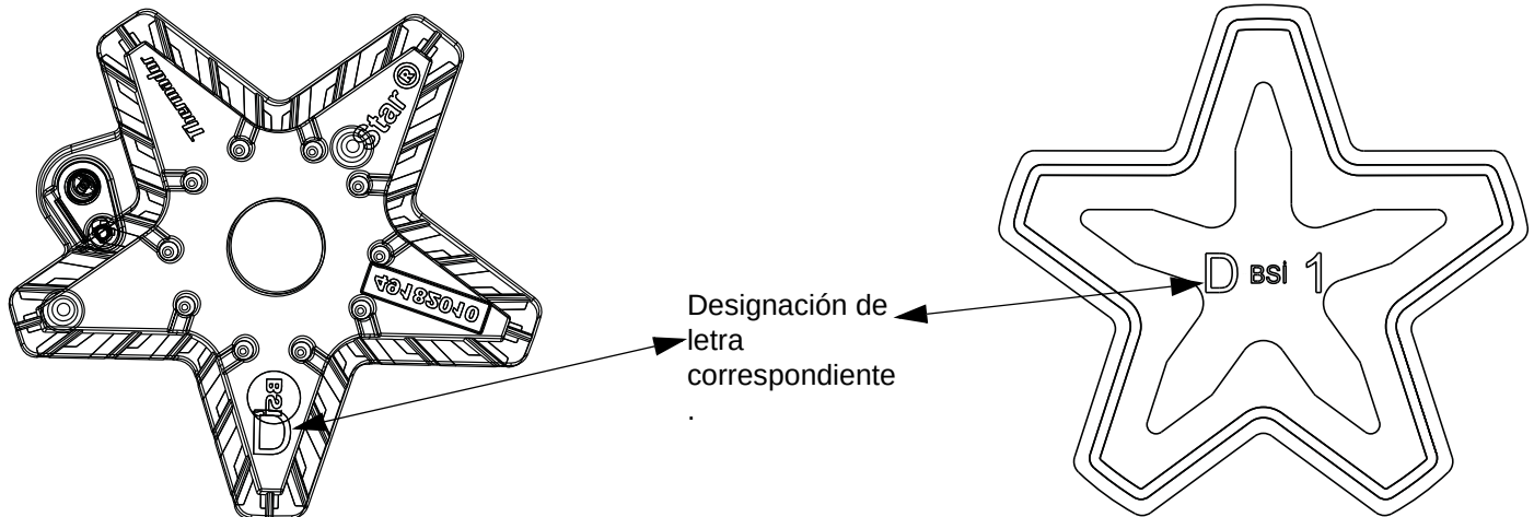
Figura 9: Tapas de las hornillas
