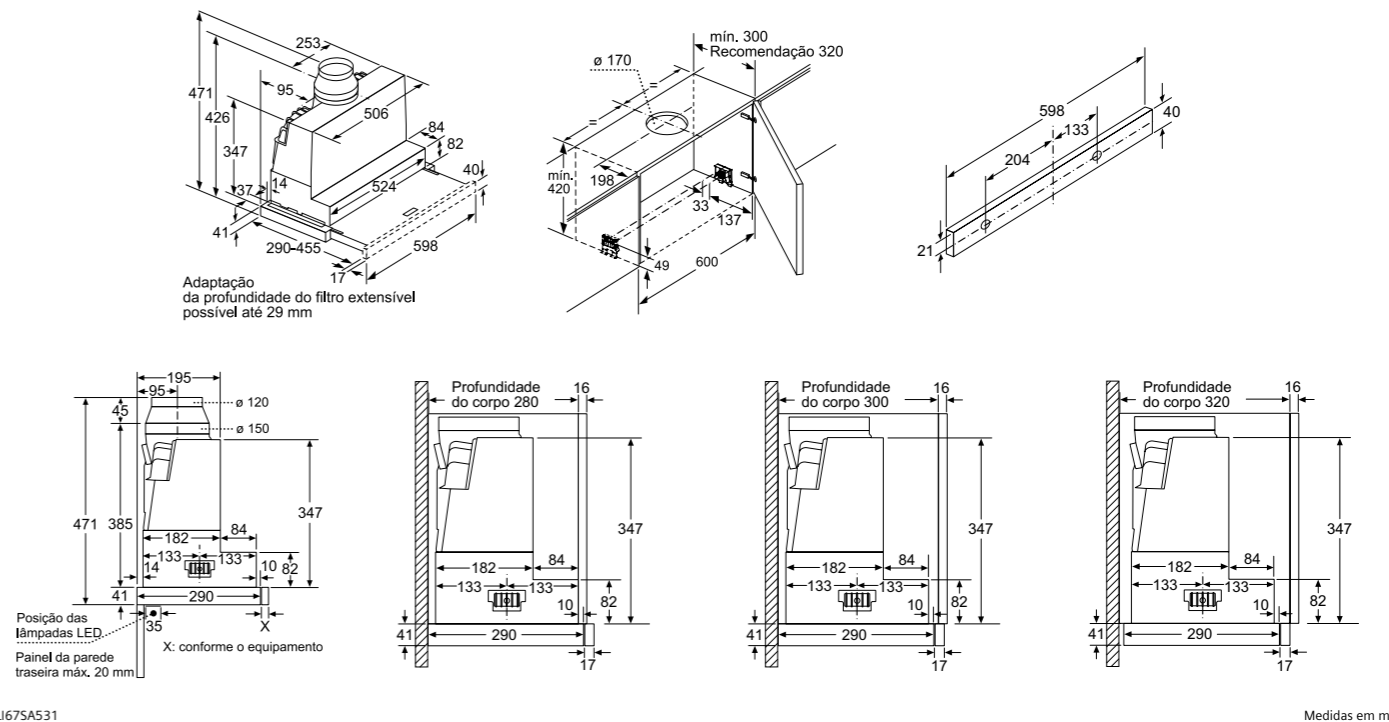
Exaustor telescópico 60 cm
